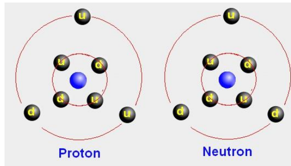
Figure 19. Hạt Proton trong nhân nguyên tử cấu tạo bởi 2 quark up + 1 quark down
