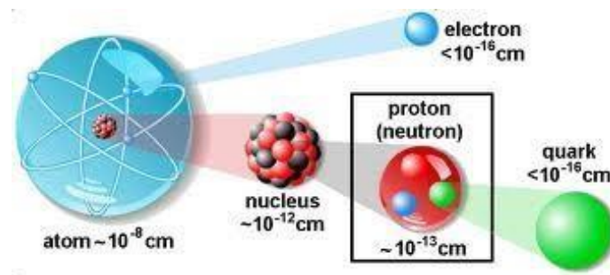
Figure 20. Size của Atom, Nucleus, Proton (Neutron), Quark and Electron
