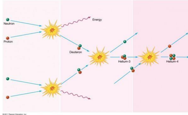
Figure 30. Những phản ứng nguyên tử, Pearson Education, Inc., 2011
