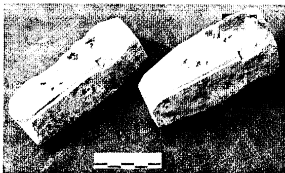
Khuôn đúc mũi tên đồng Cổ Loa (3 mang) phát hiện tại hố 3, Đền An Dương Vương
